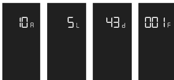
Esempio di visualizzazione per l'indirizzo fisico 10.5.43 (apparecchio n. 43, installato sulla linea 5 del campo 10) e versione firmware
