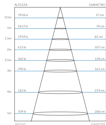
CONO DI LUCE 24° 24° CONE OF LIGHT
