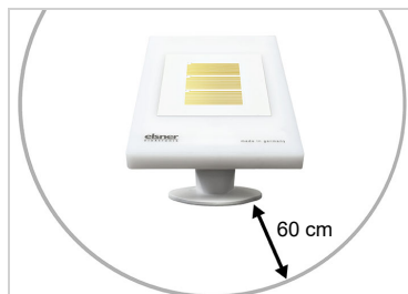
Fig. 1 Sotto, frontalmente e lateralmente, il dispositivo deve essere distante da altri elementi (elementi e parti costruttive, ecc.) almeno 60 cm.
