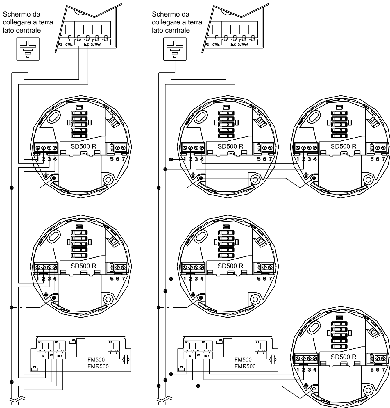
Figura 3 - Connessione dispositivi su linea aperta classe B
