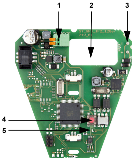
Fig. 12 1 Morsetto a molla rapido, alimentazione di tensione (20...30 V DC). Filo rigido fino a 1,5 mm 2 o filo cordato a trefoli. Assegnazione dei morsetti indipendente dalla polarità (+/- o -/+) 2 Apertura cavo alimentazione di tensione e cavo del bus 3 Connettore morsetto KNX +/- 4 Tasto di programmazione per l'apprendimento del dispositivo 5 LED di programmazione
