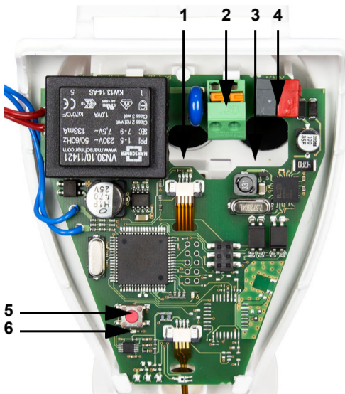
Fig. 11 1 Apertura cavo alimentazione di tensione 2 Morsetto a molla rapido, alimentazione di tensione (230 V AC), idonei per filo rigido fino a 1,5 mm 2 o filo cordato a trefoli 3 Apertura cavo alimentazione di tensione e cavo del bus 4 morsetto KNX +/- 5 Tasto di programmazione per l'apprendimento del dispositivo 6 LED di programmazione
