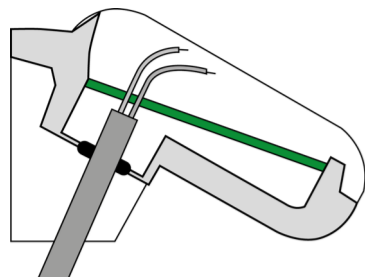
Fig. 10 Posizionare la guaina del cavo sotto la scheda e far passare solo il cavo di collegamento attraverso i fori della scheda verso alto.
