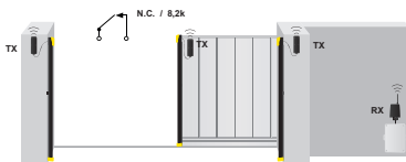
Portail coulissant
