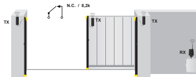
Automatisierung Schiebetor
