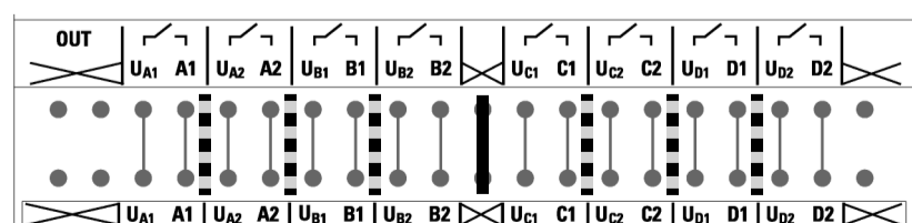
Fig. 4 Caratteristiche di isolamento dei gruppi di morsetti ■ ■ ■ Isolamento 6 kV (rinforzato) - - - Isolamento 4 kV (semplice)
