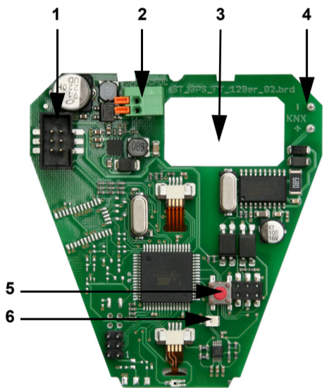
Fig. 13 1) Connettore della connessione a cavo per il sensore precipitazioni sul coperchio della scatola 2) Morsetto a molla rapido, alimentazione di tensione (20...30 V DC). Filo rigido fino a 1,5 mm 2 o filo cordato a trefoli. Assegnazione dei morsetti indipendente dalla polarità (+/- o -/+) 3) Apertura cavo alimentazione di tensione e cavo del bus 4) Connettore morsetto KNX +/- 5) Tasto di programmazione per l'apprendimento del dispositivo 6) LED di programmazione
