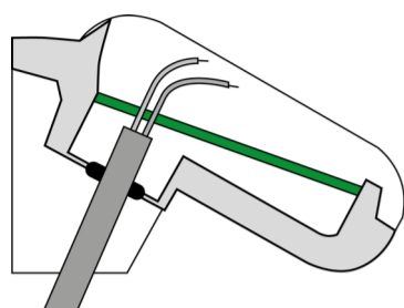
Fig. 11 Posizionare la guaina del cavo sotto la scheda e far passare solo il cavo di collegamento attraverso i fori della scheda verso alto.
