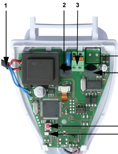
Fig. 12 1) Connettore per il sensore precipitazioni sul coperchio della scatola 2) Apertura cavo alimentazione di tensione 3) Morsetto a molla rapido, alimentazione di tensione (230 V AC), idonei per filo rigido fino a 1,5 mm 2 o filo cordato a trefoli 4) Connettore per morsetto KNX +/- 5) Apertura cavo del bus 6) Tasto di programmazione per l'apprendimento dell'apparecchio 7) LED di programmazione
