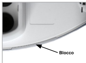
Fig. 14 Verificare il perfetto incastro del coperchio nella parte inferiore! La figura mostra l'alloggiamento chiuso da sotto.
